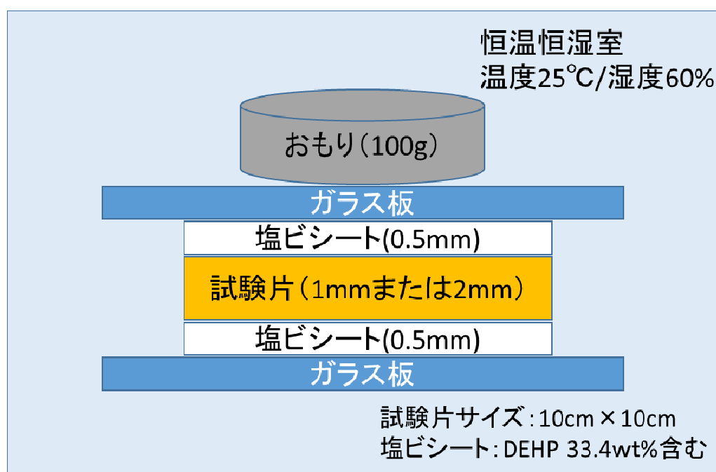
図2 接触移行性試験の条件
