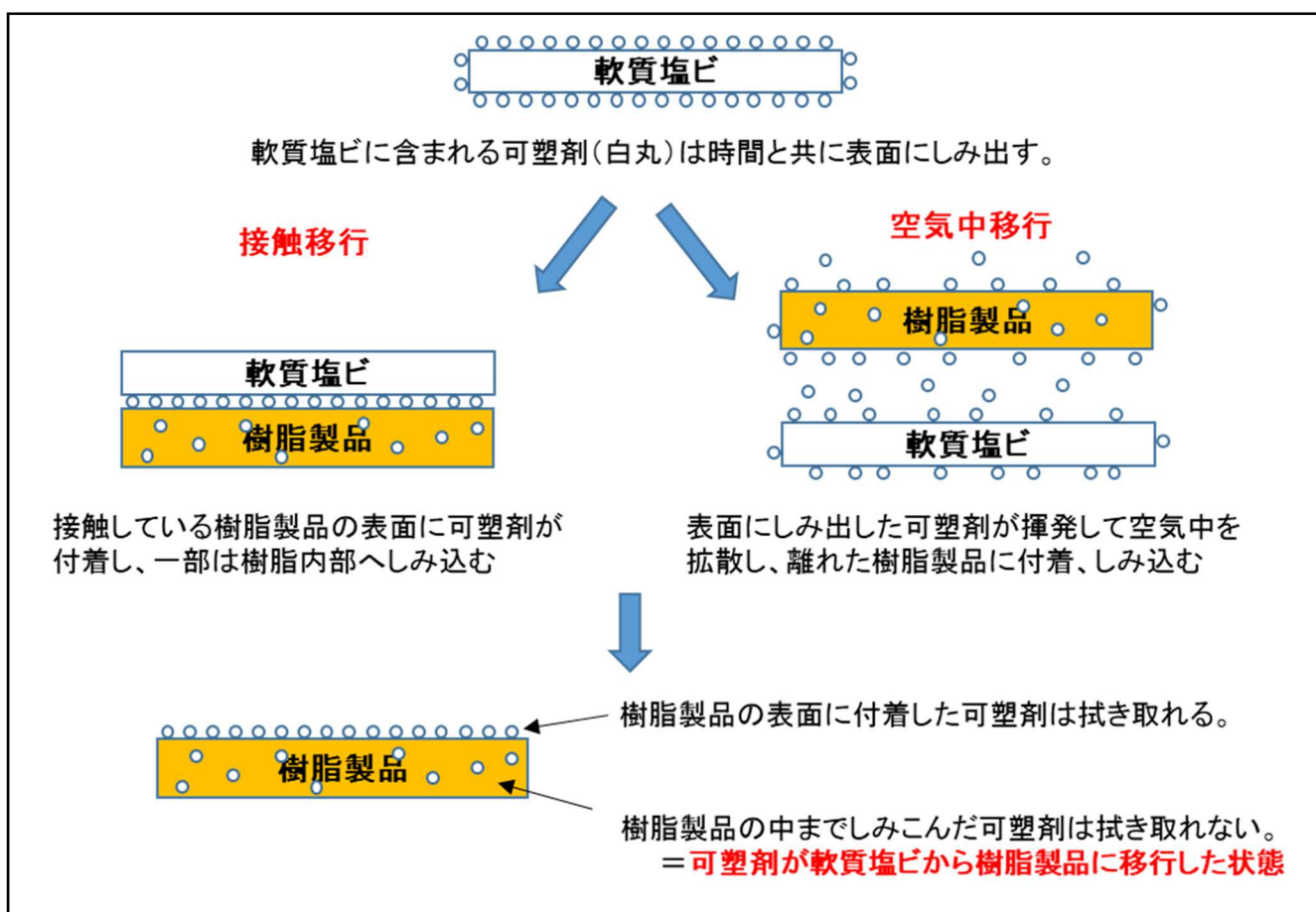
図1 可塑剤が移行する状態とは
